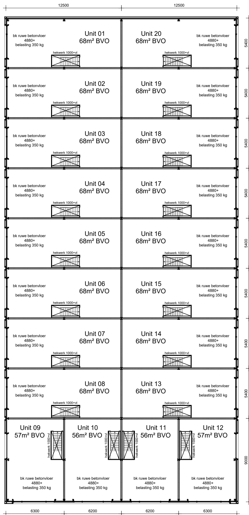
1e Verdieping
